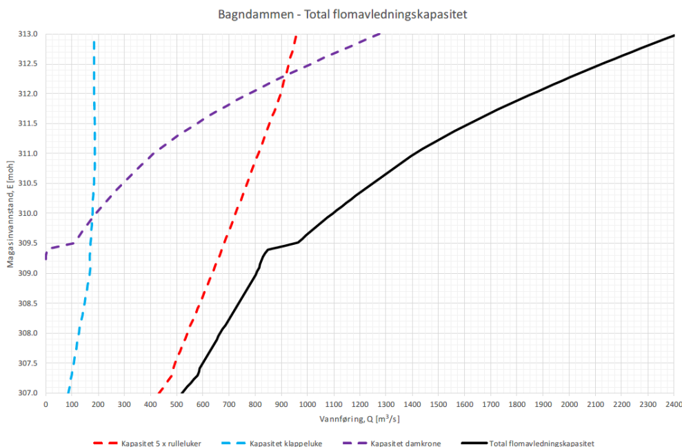
Figur 3 Kapasitetskurve Bagndammen (fra flomberegninger Bagndammen 2020, NN1954).
