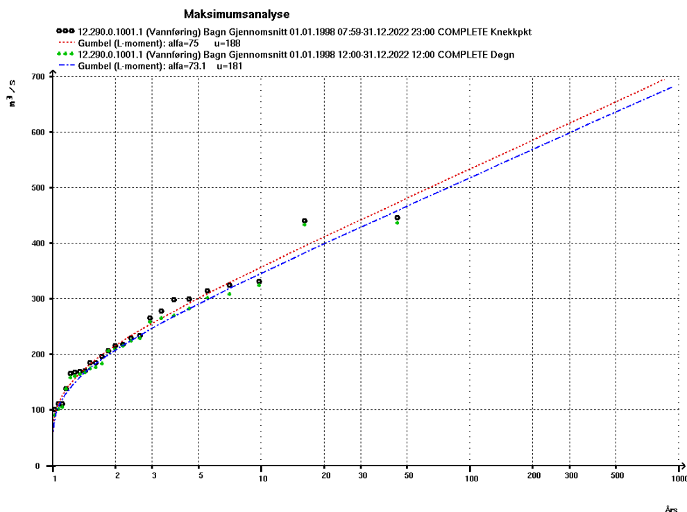
Figur 10 Frekvensanalyse på døg- og knekkpunktdata fra 12.290 Bagn. 1998-2022.
