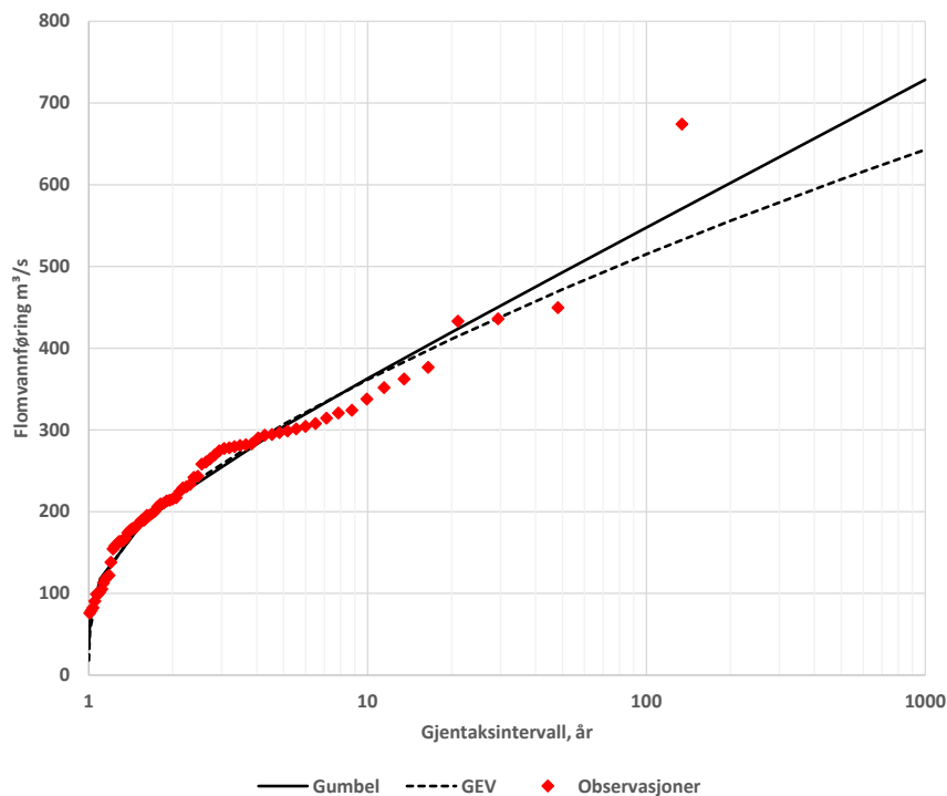
Figur 8 Flomfrekvensanalyse på årlige høyeste vannføringer ved 12.290 Bagn. Periode 1949-2023.
