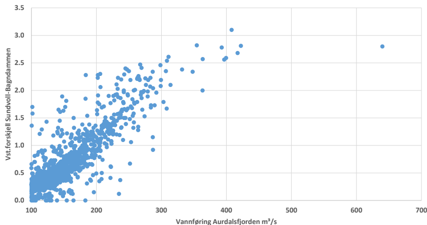
Figur 5 Observert vannstandsforskjell mellom Sundvoll og Bagndammen (1965-2017+2023).
